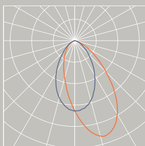
EN Lighting result with a 20° adjustment of the product IT Resa illuminotecnica con il prodotto posizionato a 20°
