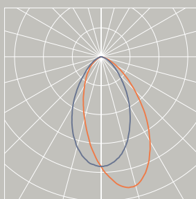
EN Lighting result at 10° adjustment of the product IT Resa illuminotecnica con il prodotto posizionato a 10°
