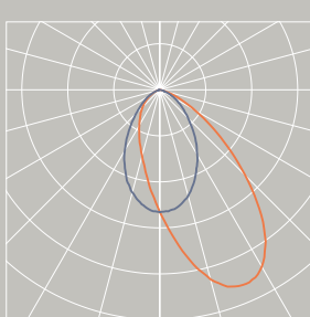
EN Lighting result with a 30° adjustment of the product IT Resa illuminotecnica con il prodotto posizionato a 30°
